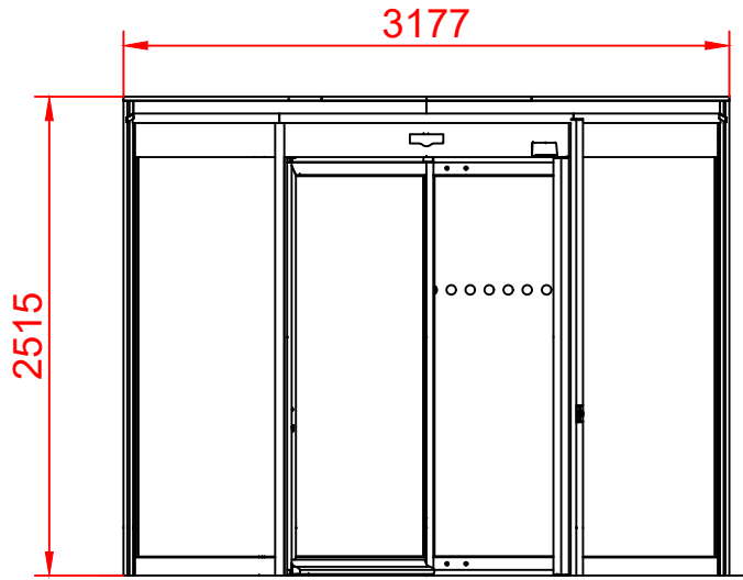
ÖRNEK 3000mm 3 KANAT DÖNER KAPI
