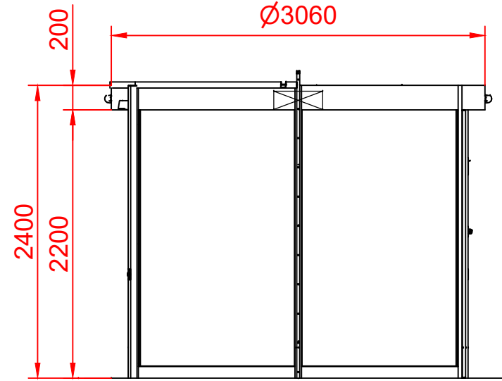
ÖRNEK 3000mm 3 KANAT DÖNER KAPI
